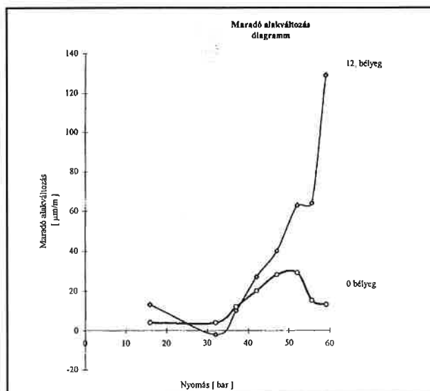
9/b. ábra A kivágás sarkába telepített, legnagyobb alakváltozást regisztrált (12. jelű) bélyeg és a referencia (0. jelű) bélyeg által mért maradó alakváltozások
